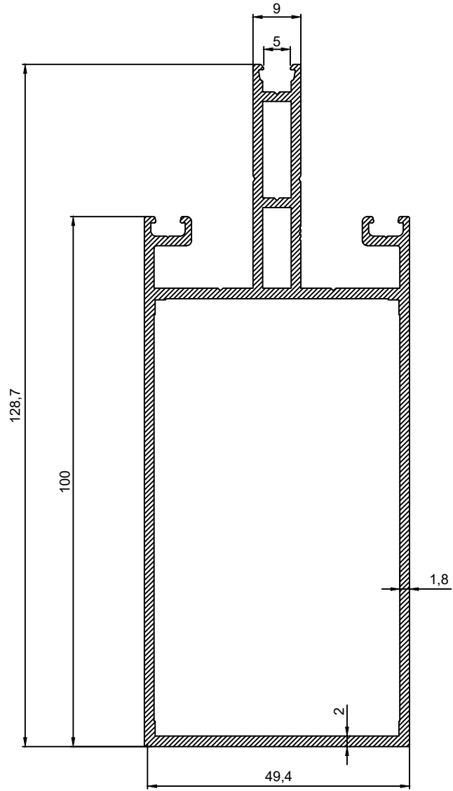
P.No 15089 2.033 Kg/m
