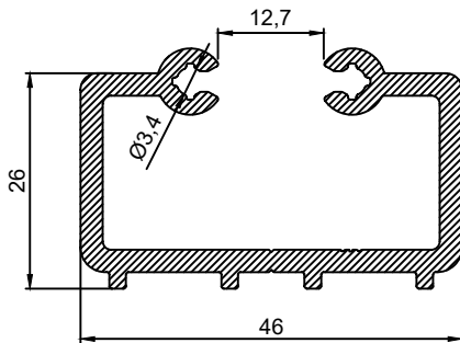
P.No 15092 0.951 Kg/m
