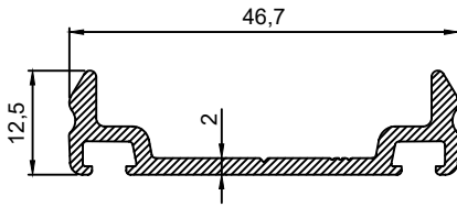
P.No 15091 0.409 Kg/m
