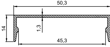
P.No 15090 0.285 Kg/m
